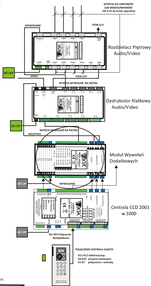
SCHEMAT BLOKOWY SYSTEMU CCD 2001 w.1000
