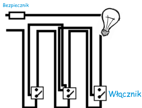
Instalacja tradycyjna schodowa
